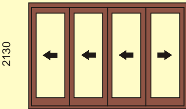
4 Door 2556 3359 Width
