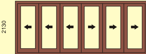
6 Door 3785 4985 Width
